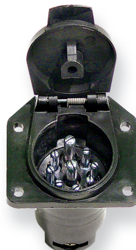
▲ Boom Pendant Outlet 631-0192 (9 Pin) 631-0005 (8 Pin)
