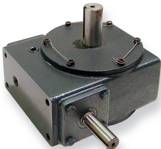
▲ Boom Gear Box 646-0035
